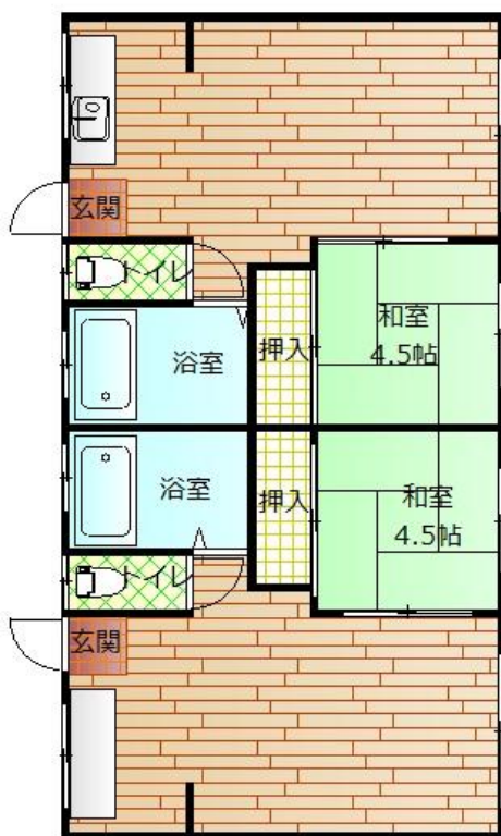
1階平面図
