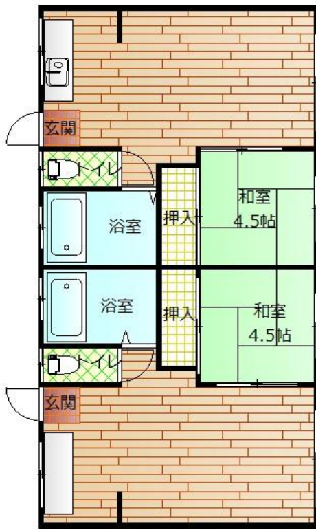
1階 平面図
